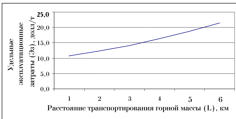
Рис. 4. Зависимость удельных эксплуатационных затрат от расстояния транспортирования горной массы
