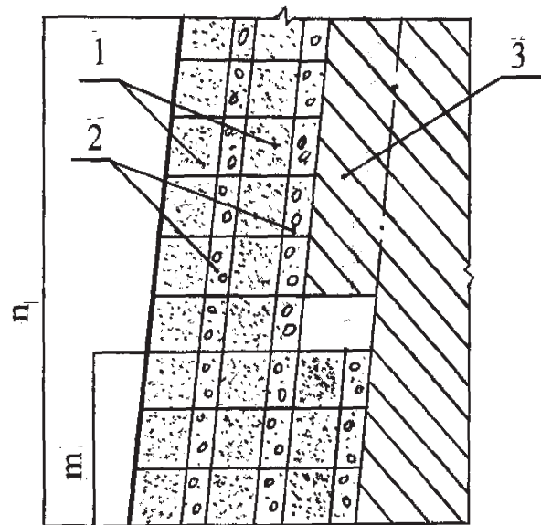
Рис. 2. Схема комбинированной закладки выработанных пространств очистных слоев при выемке наклонных прирезок: 1 – бетонные стенки; 2 – гранулированная закладка в отработанных слоях; 3 – наклонные прирезки
