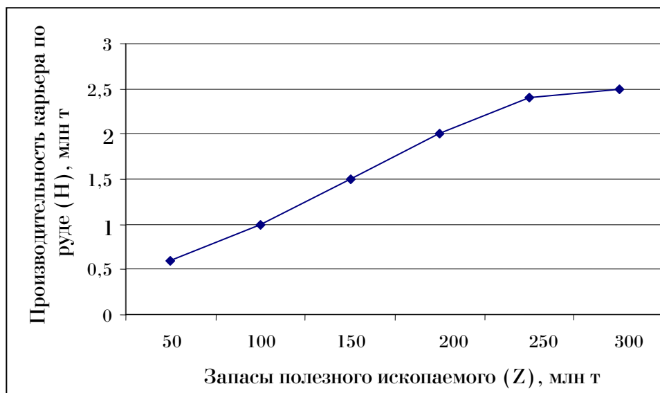
Рис. 3. Зависимость производительности карьера по руде от величины запасов полезного ископаемого в его контуре
