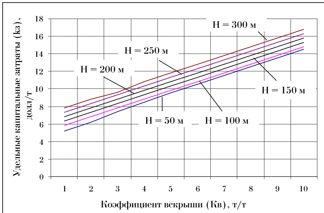
Рис. 1. Зависимость удельных капитальных затрат от коэффициента вскрыши и глубины карьера
