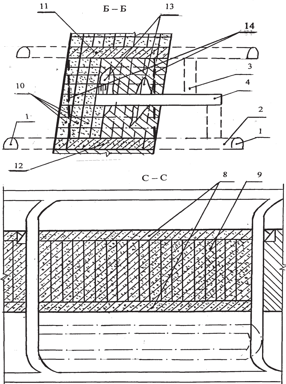
Рис. 1. Система разработки крутопадающих сложных мощных рудных тел сплошной слоевой выемкой наклонных прирезок с закладкой
