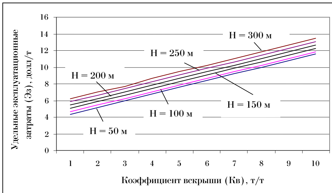
Рис. 2. Зависимость удельных эксплуатационных затрат от коэффициента вскрыши и глубины карьера
