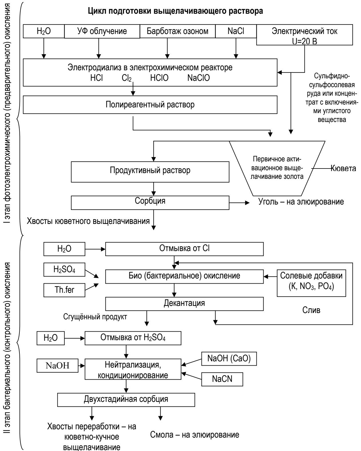
Рис. 2. Схема лабораторных экспериментальных исследований комбинированных методов окисления сульфидно-сульфосолевой золотосодержащей руды или концентрата (с углистыми включениями)
