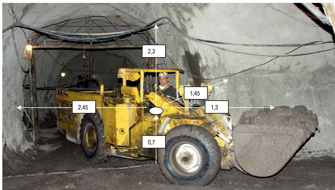
Рис. 5. Расстояния от центра сидения оператора ПДМ ПД-2Э до излучающих участков очистной выработки и центра ковша
