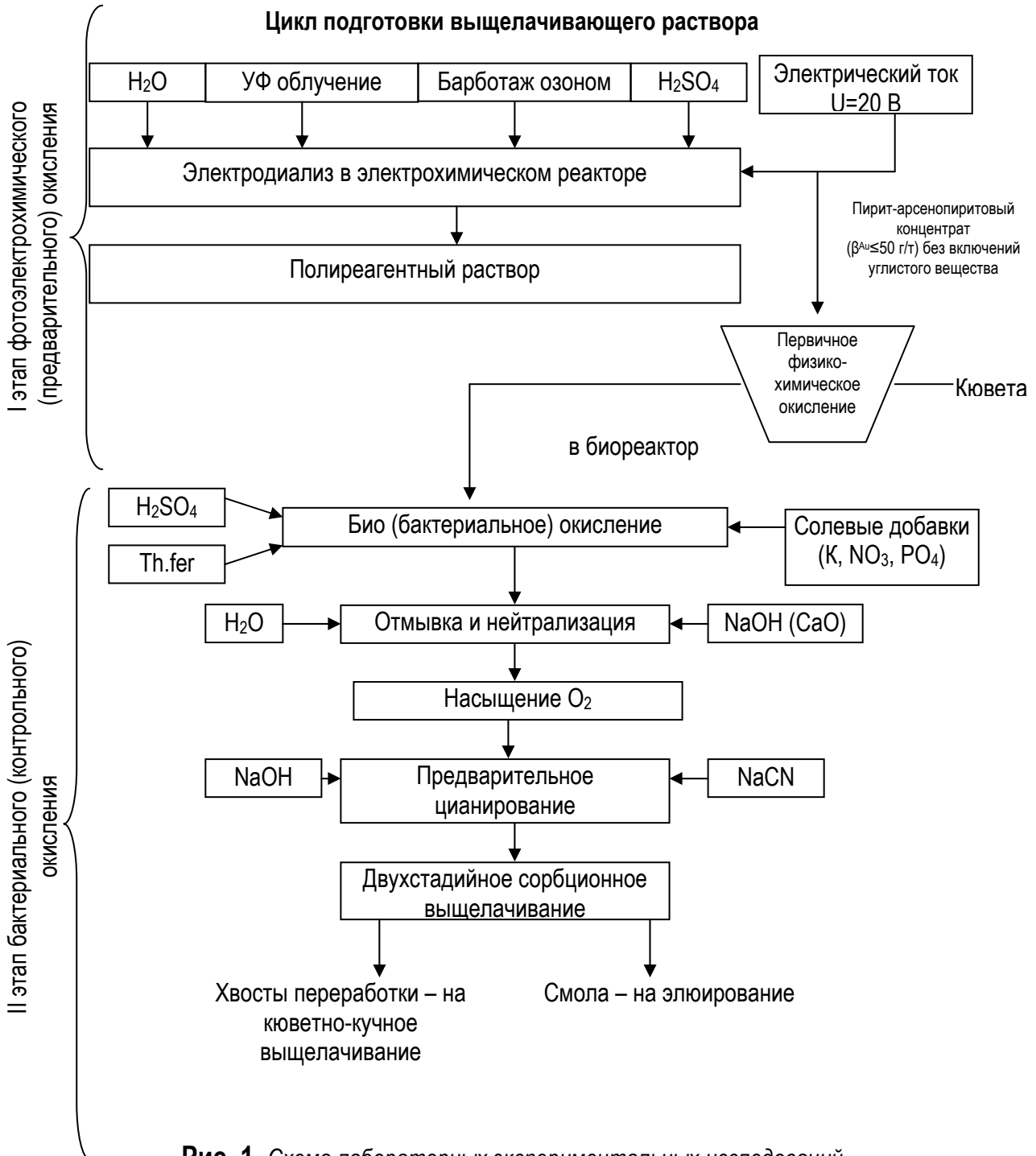
Рис. 1. Схема лабораторных экспериментальных исследований комбинированных методов окисления
