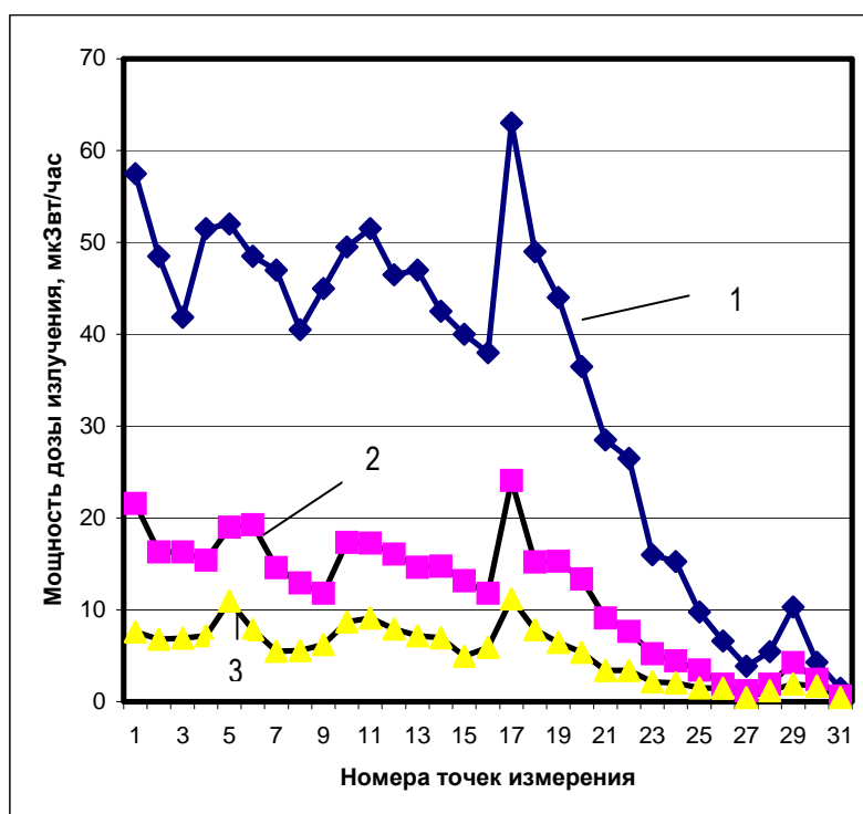
Рис. 2. Уровень радиации в блоке 5-704:
