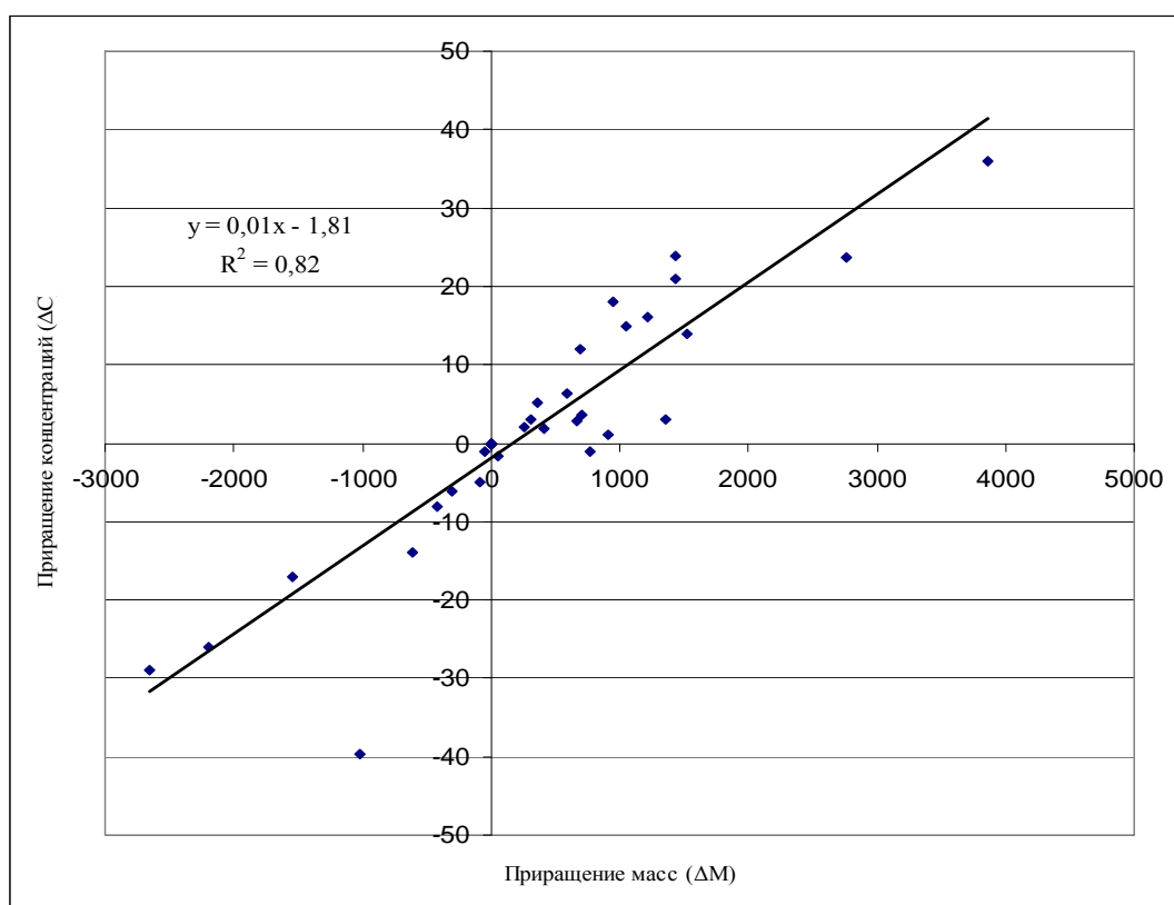
Рис. 2. Зависимость изменения содержания марганца от концентрации в начальном и конечном створах по длине р. Ингода в Забайкальском крае
