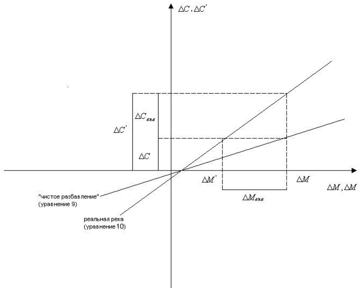
Рис. 3. Схема соотношения изменения масс химического вещества или соединения в русле реальной реки и для случая «чистого разбавления» (индексы i, i+1, j у обозначений опущены)
