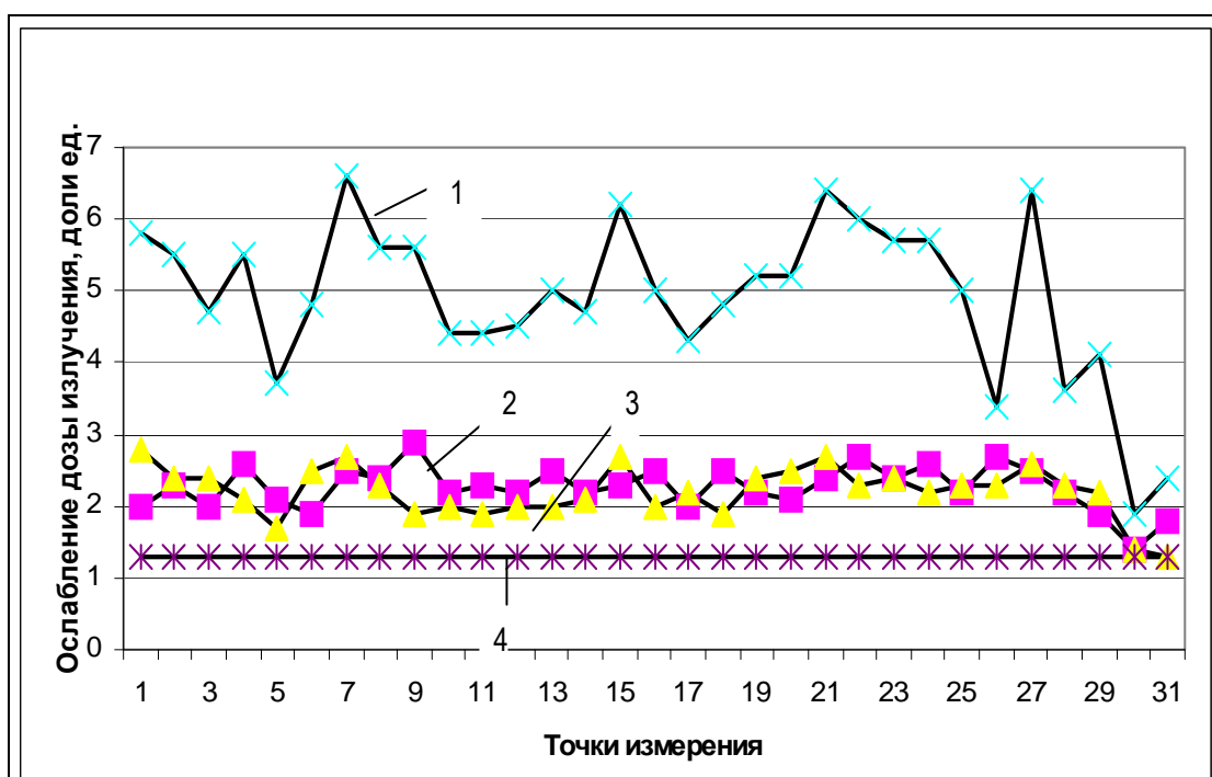
Рис. 3. Кратность ослабления дозы излучения: 1 – телом человека; 2 – ПДМ; 3 – защитой из свинцового листа толщиной 10 мм; 4 – ПДМ с защитой из свинцового листа толщиной 10 мм
