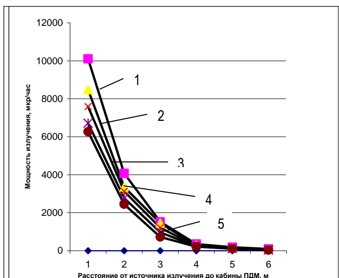
Рис. 1. Зависимость интенсивности излучения от расстояния между источником и кабиной ПДМ:
