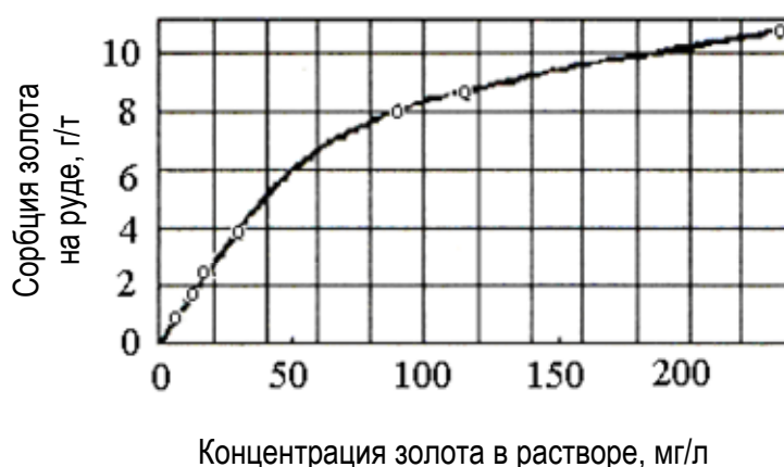
Изотерма сорбции цианида золота на руде крупностью -10 мм
