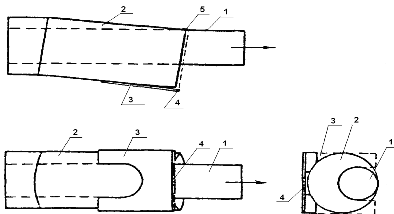
Рис. 4. Коаксиальная аэродинамическая насадка:
