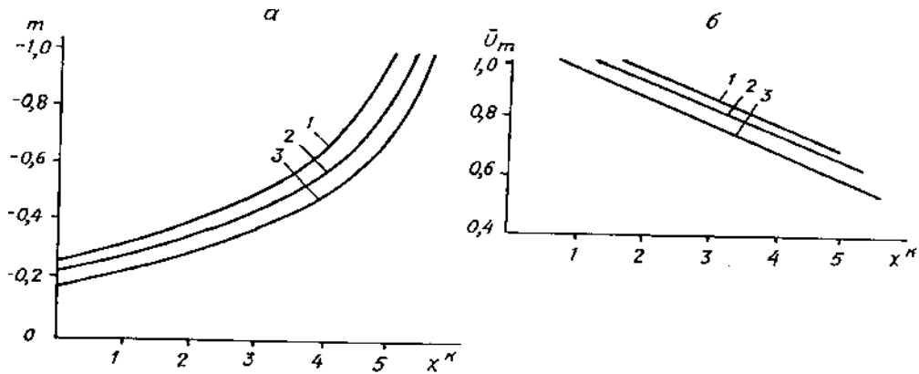
Рис. 3. Изменение безразмерной скорости встречного потока (а) осевой скорости струи (б) по длине призабойной зоны выработки \rho : 1 – 1,0; 2 – 0,8; 3 – 0,6
