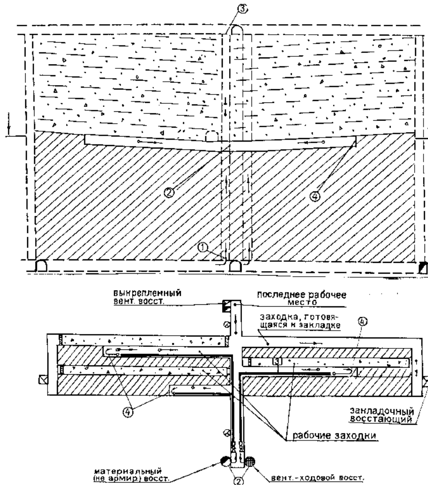
Рис. 1. Рациональная схема проветривания очистного блока при слоевой системе разработки с нисходящей выемкой и твердеющей закладкой
