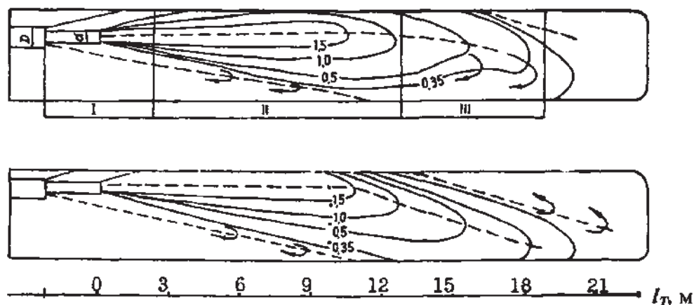
Рис. 5. Структура вентиляционной струи в призабойной зоне для коаксиальной насадки
