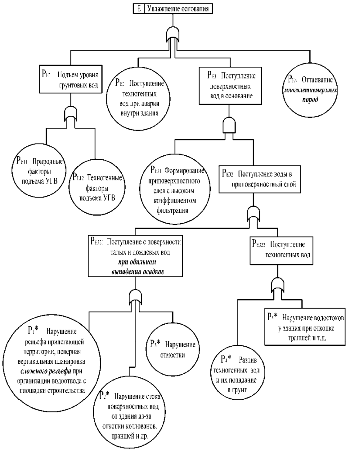
Рис. 2. Дерево отказов. Фрагмент E
