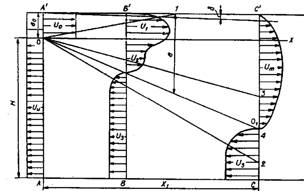
Рис. 2. Схема распространения струи во встречном потоке 1-4 – направления распространения струи
