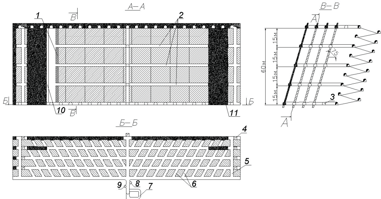
Рис. 3. Система разработки подэтажных штреков со сплошной выемкой с последующим заполнением выработанного пространства твердеющей закладкой: 1 – взрывные скважины; 2 – подэтажный штрек; 3 – транспортный штрек; 4 – вентиляционно-ходовой восстающий; 5 – орт-заезд; 6 – погрузочный орт-заезд; 7 – спиральный съезд; 8 – вентиляционный восстающий; 9 – рудоспуск; 10 – отрезной восстающий
