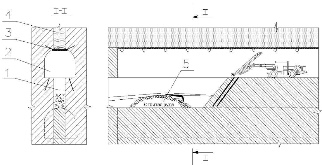
Рис. 2. Технологическая схема отработки слоя (вариант № 2): 1 – щель; 2 – слой; 3 – крепь; 4 – щель, заполненная твердеющей закладкой; 5 – отбитая руда
