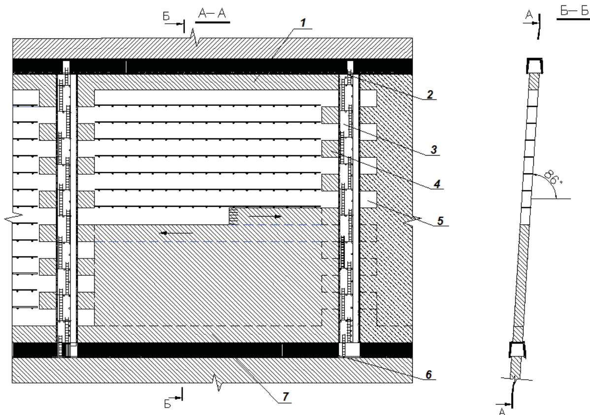
Рис. 4. Система разработки с нисходящей слоевой выемкой и креплением выработанного пространства:
