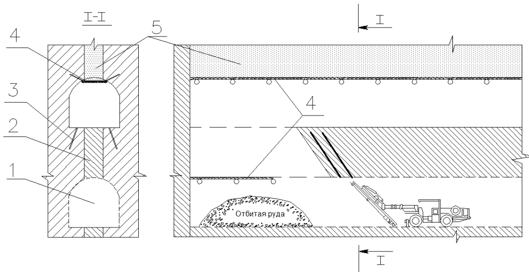
Рис. 1. Технологическая схема отработки слоя: 1 – очистная заходка; 2 – щель; 3 – анкерная крепь; 4 – защитная крепь; 5 – щель, заполненная твердеющей закладкой
