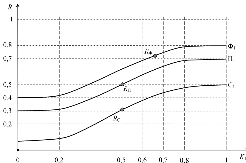
Рис. 2. Изолинии K_2 = \text{const} поверхности вывода R = f(K_1, K_2) : K_2=0,718(\Phi_1) , K_2=0,5(\Pi_1) , K_2=0,215(C_1) Fig. 2. Surface R = f(K_1, K_2) isolines K_2 = \text{const} : K_2=0,718(\Phi_1) , K_2=0,5(\Pi_1) , K_2=0,215(C_1)
