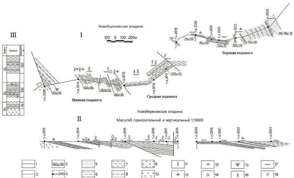
Рис. 2. Новоберёзовский гипостратотип-1. I – абрис укурейской свиты; II – геологический разрез укурейской свиты; III – стратиграфическая колонка. Условные обозначения: 1 – тектонические нарушения; 2 – границы слоев; 3 – элементы залегания; 4 – номера точек наблюдения; 5 – песчаники; 6 – алевролиты; 7 – аргиллиты; 8 – частое переслаивание песчаников и алевролитов; 9 – туфопесчаники; 10 – эффузивы. Органические остатки: 11 – насекомые; 12 – растения; 13 – щитни; 14 – линцеусы; 15 – чекановские; 16 – хвощи; 17 – следы илоедов; 18 – следы феррофибры
